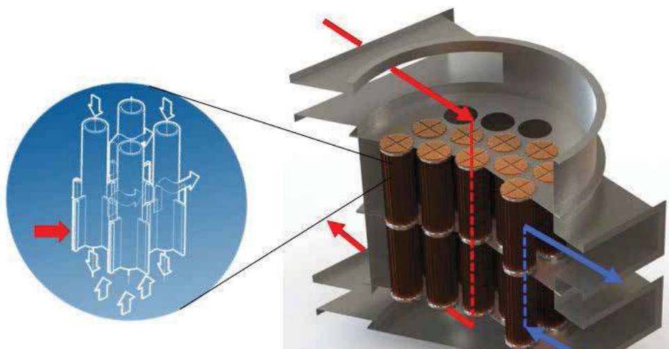
»3 HeatMatrix Luvu gas exchanger »3 HeatMatrix Gas-Tauscher
